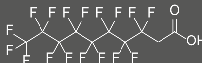
8:2 FTCA; H2PFDA
